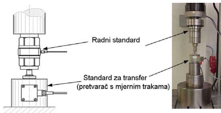
Slika 3. Standardna procedura kalibracije [3]
